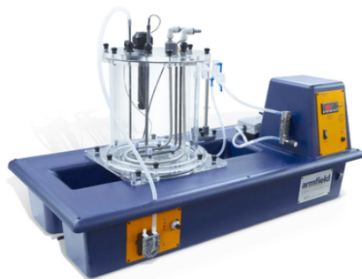
DIGESTORE AEROBICO
